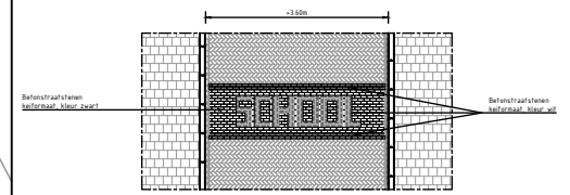
Detail 1: SCHOOL-markering wegbreedte groter dan 3,50m Schaal 1:100
