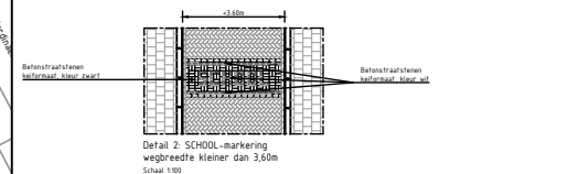
Detail 2: SCHOOL-markering wegbreedte kleiner dan 3,50m Schaal 1:100
