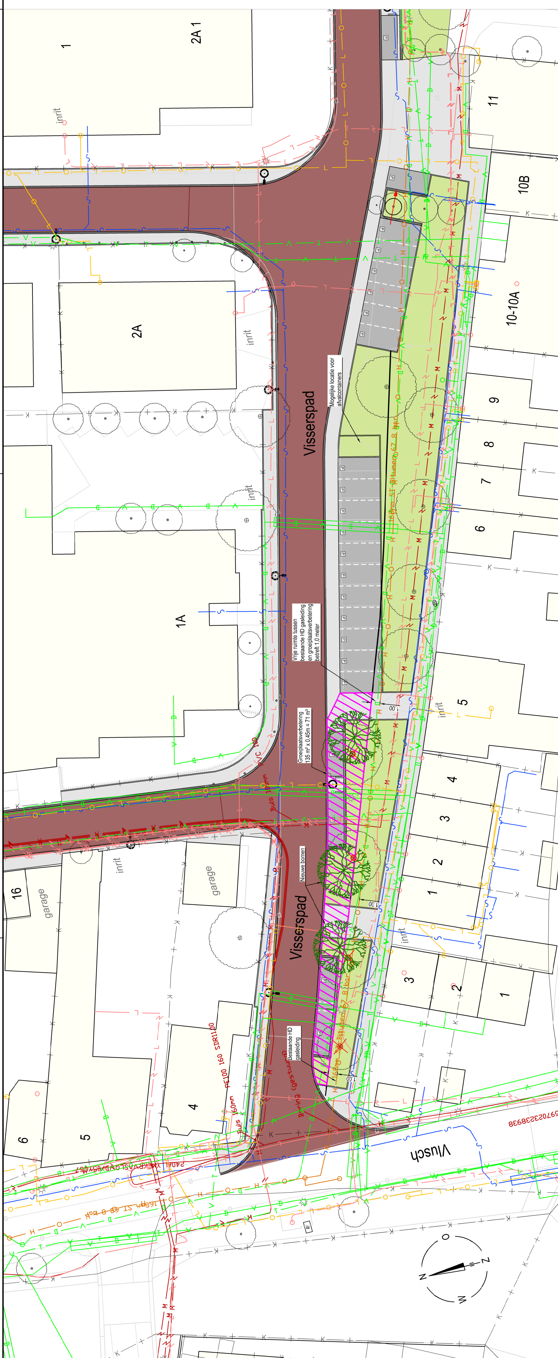
Situatieoverzicht Schaal 1:250
