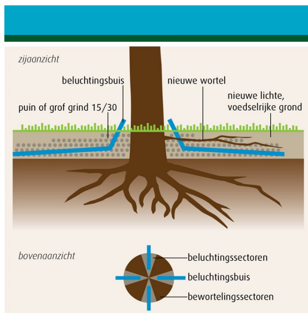
Figuur 10 beluchting bij grondophoging
